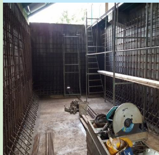
• Travaux en cours : Vue intérieure de l'un des compartiment du filtre à sable. Avec ses nouvelles armatures il devrait être plus résistant.
